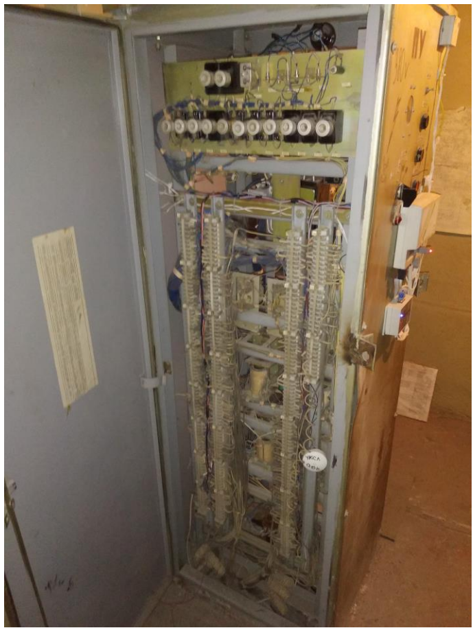
Рисунок 5– Шкаф управления
