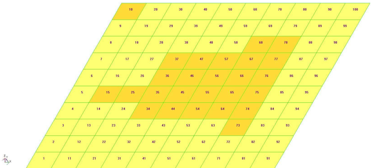
Площадь арматуры на 1м² по оси Y у нижней грани (балки-стены - посередине), максимум в элементе 65
