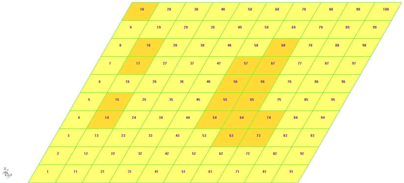
Площадь арматуры на 1м² по оси X у нижней грани (балки-стены - посередине), максимум в элементе 65
