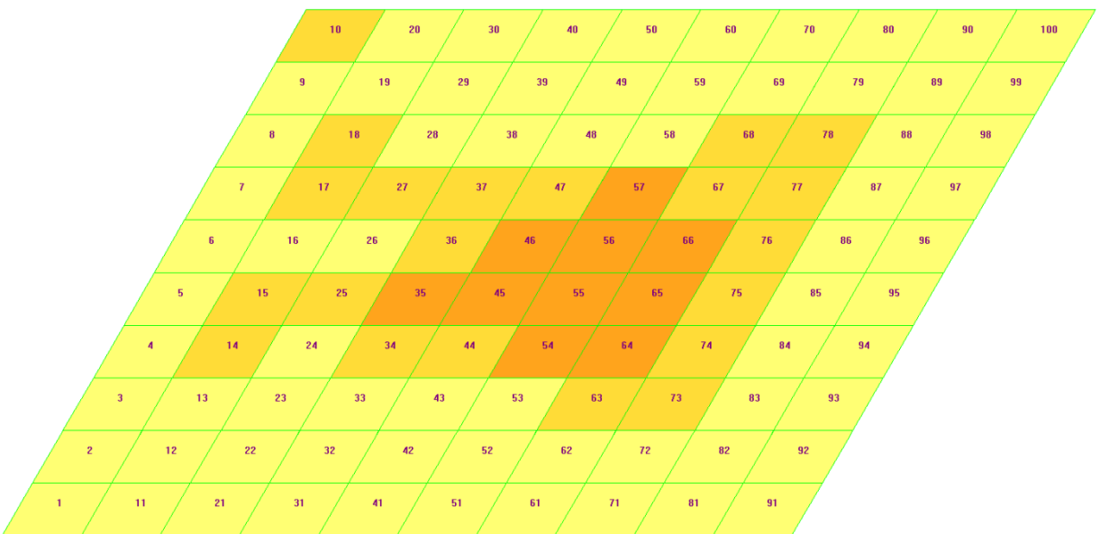
Рис. 6. Площадь арматуры на 1 пог. м по оси Y по нижней грани.
