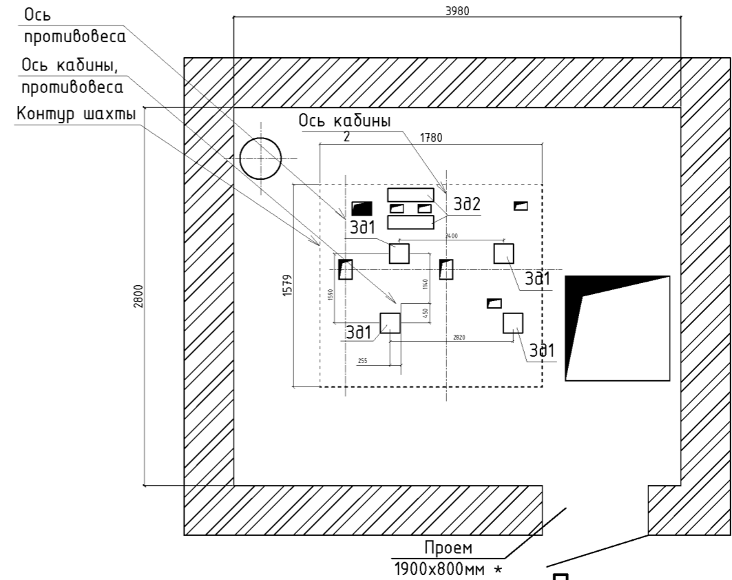
План приямка.
